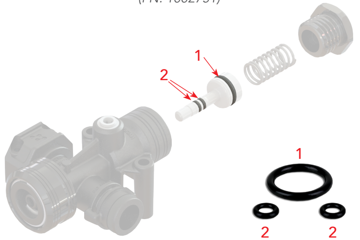
MAM O-RING REPAIR KIT (PN: 1002751)
